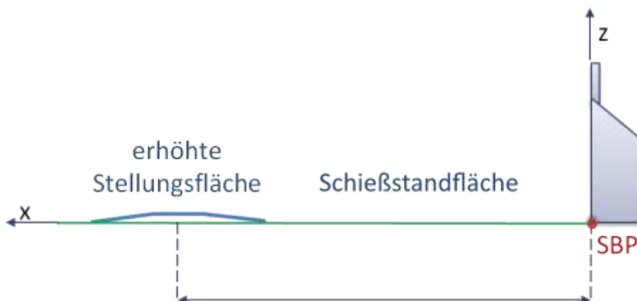
Abbildung 7 Skizze zum Bezugssystem im Schießstandtyp D Darstellung in der Schießstandmittelebene Schießrichtung von links nach rechts
